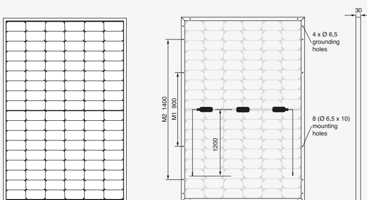
Abb. Prinzipskizze
